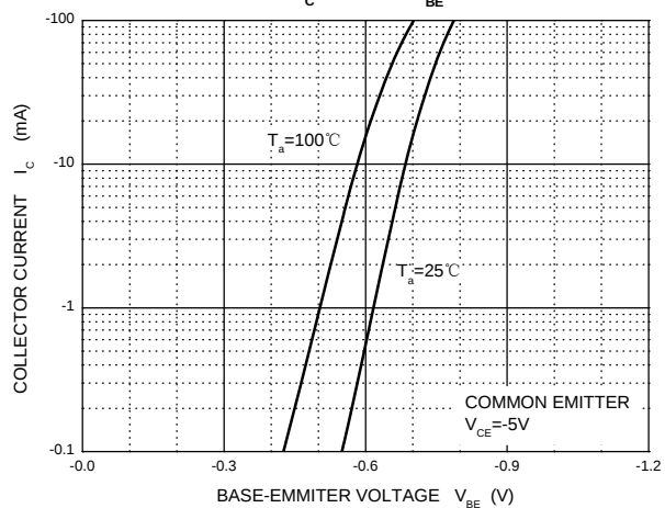
I_C — V_{BE}
