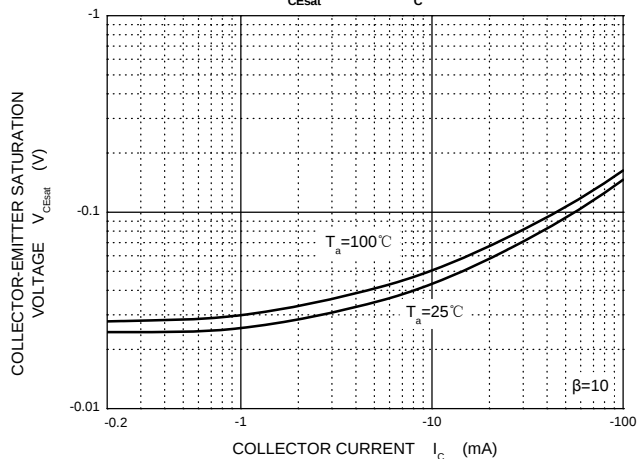
V_{CEsat} — I_C
